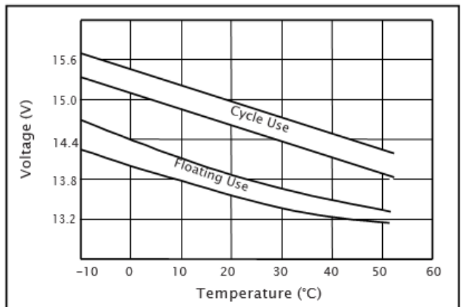
Зарядное напряжение при температуре
